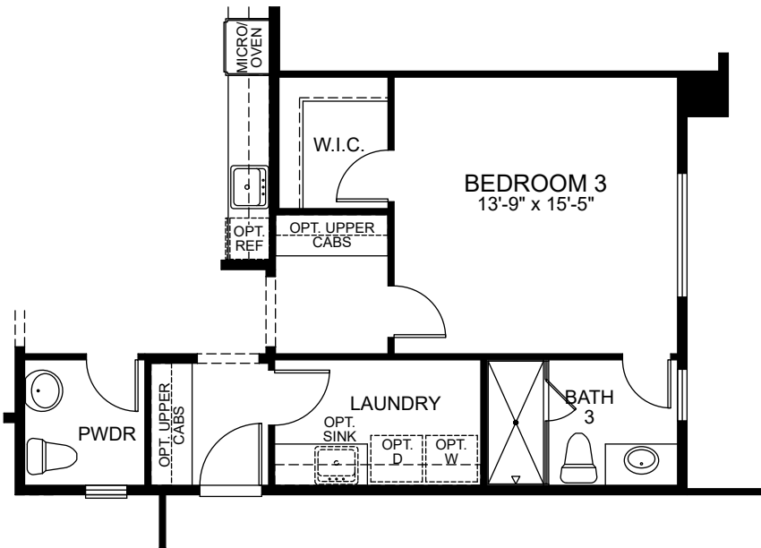
OPT. BEDROOM SUITE 3
